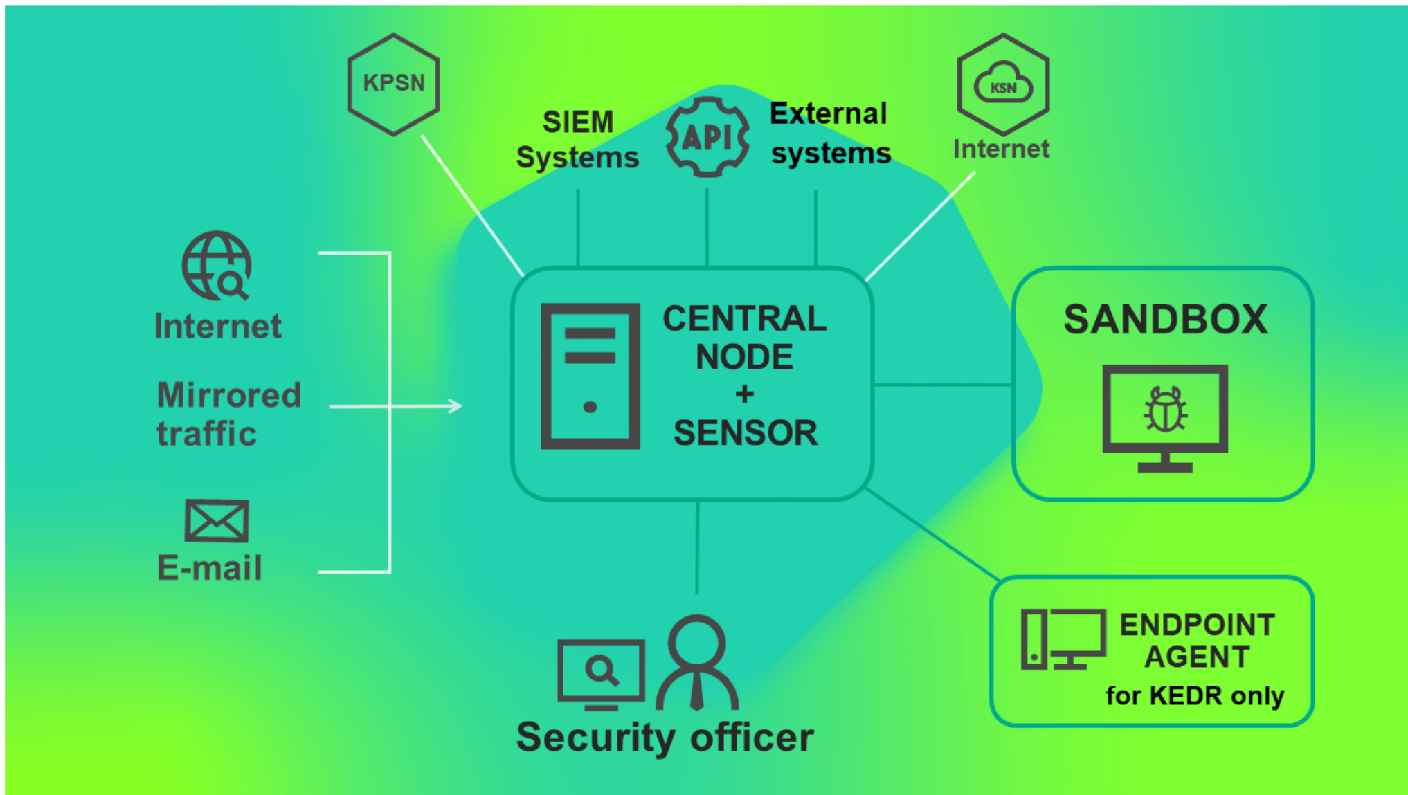
Схема работы приложения при развертывании на два сервера
