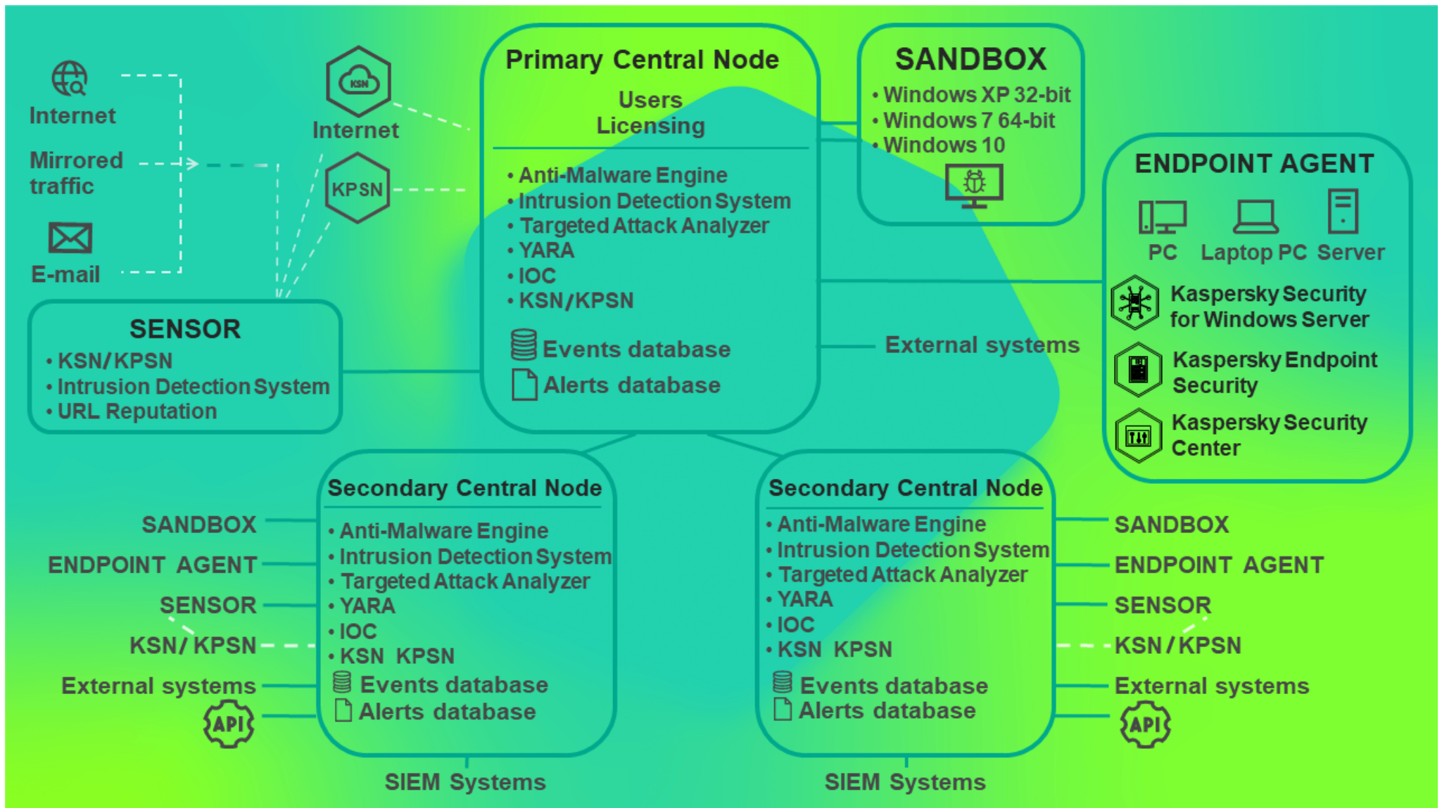
Принцип работы приложения в режиме распределенного решения
