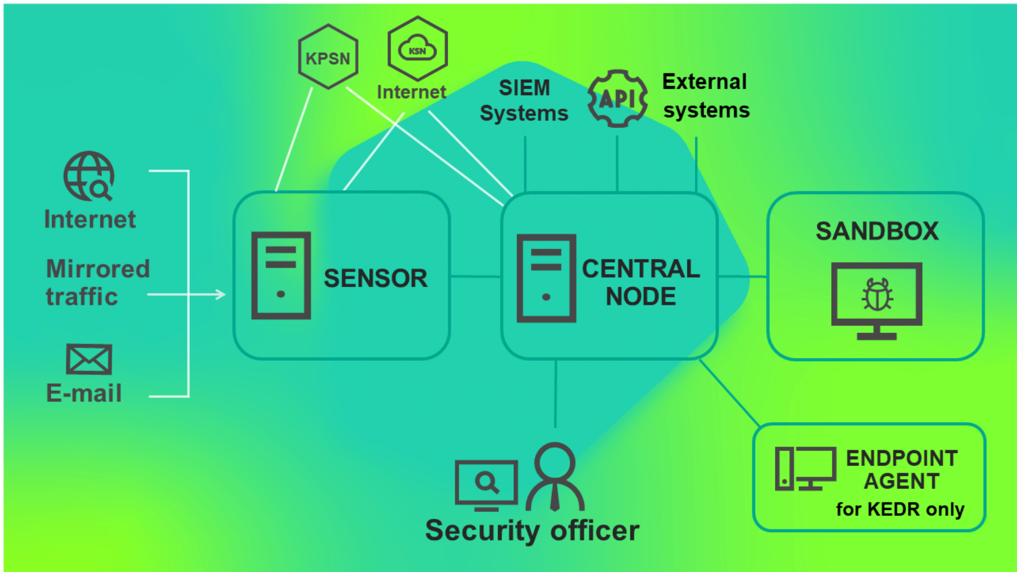
Схема работы приложения при развертывании на три сервера
