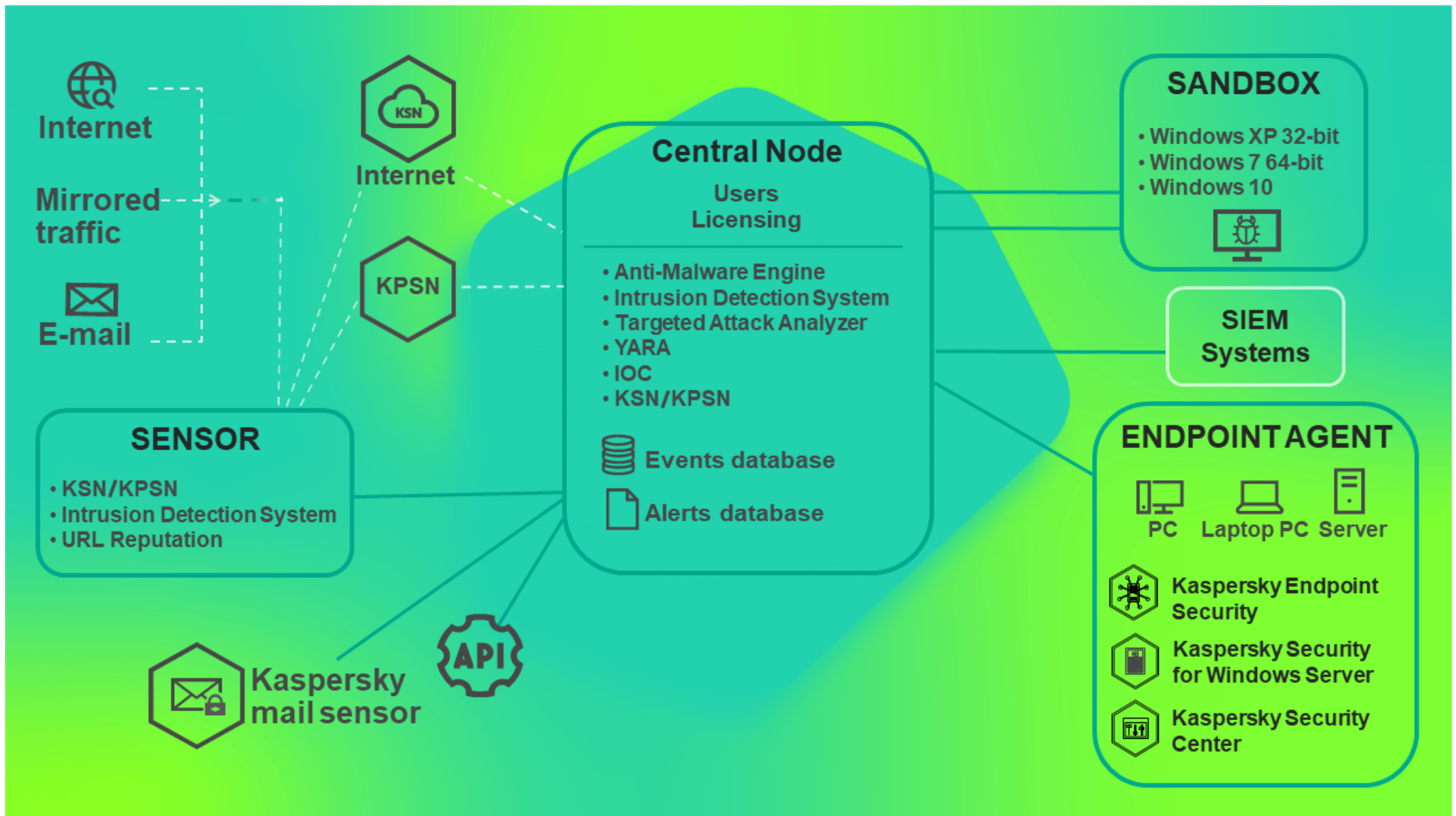
Принцип работы Kaspersky Anti Targeted Attack Platform
